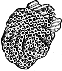
चित्र १५—सिलूरियन काल का मूँगा
